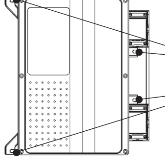
Position des 4 trous pour la fixation du boîtier sur un plan.
